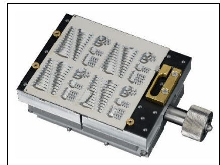
4x4" Substrataufnahme m. gummierter Oberfläche, mit mechanische Klemmung
